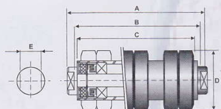
ROLETE DE GUIA - CÓD.: N. RG130
