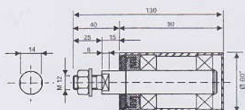
ROLETE DE GUIA - CÓD.: N. RG130
